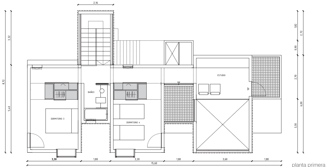
planta primera
