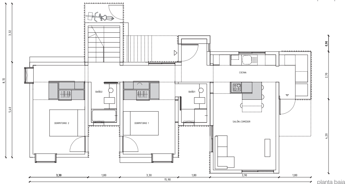
planta baja
